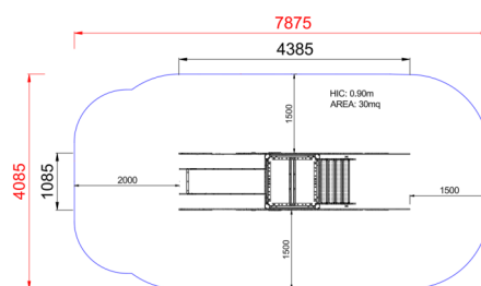
Area di sicurezza totale / Total safety area: 30mq Altezza Max di Caduta / Max falling height: 0.90m
