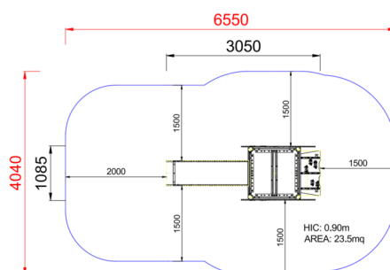
Area di sicurezza totale / Total safety area: 23.5mq Altezza Max di Caduta / Max falling height: 0.90m
