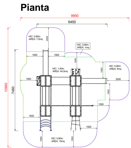
Area di sicurezza totale / Total safety area: 77mq Altezza Max di Caduta / Max falling height: 1.40m
