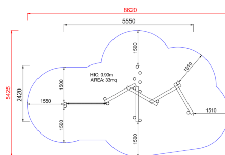
Area di sicurezza totale / Total safety area: 33mq Altezza Max di Caduta / Max falling height: 0.90m
