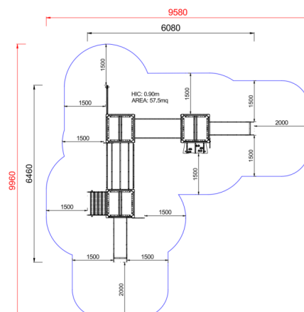
Area di sicurezza totale / Total safety area: 57.5mq Altezza Max di Caduta / Max falling height: 0.90m
