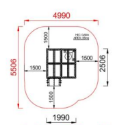
Area di sicurezza totale / Total safety area: 25mq Altezza Max di Caduta / Max falling height: 0.60m
