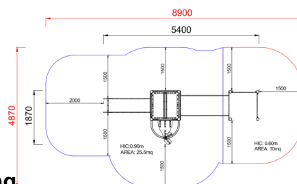
Area di sicurezza totale / Total safety area: 35.5mq Altezza Max di Caduta / Max falling height: 0.90m
