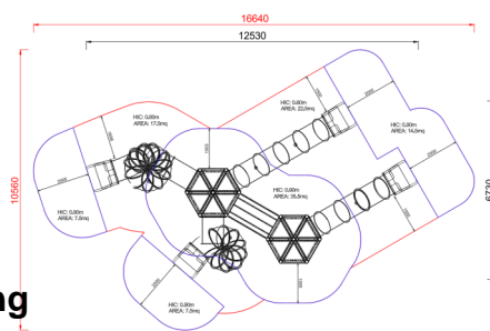
Area di sicurezza totale / Total safety area: 105mq Altezza Max di Caduta / Max falling height: 0.90m
